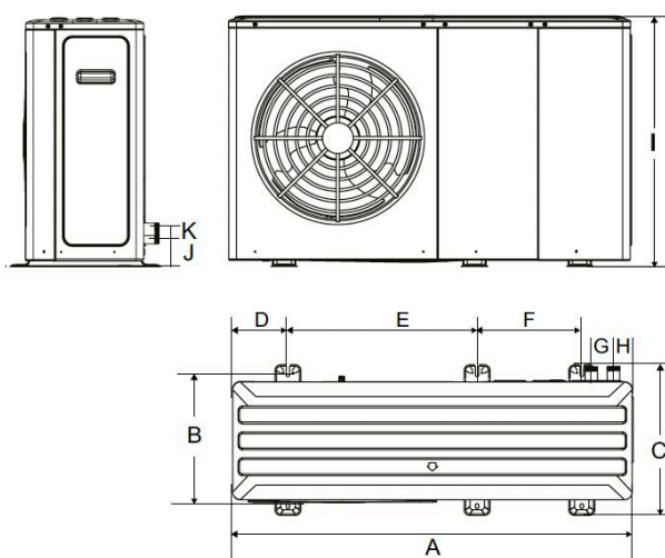
8/10/12/14/16 kW (unidad:mm)
