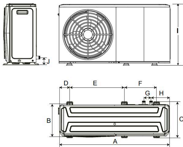
4/6 kW (unidad:mm)
