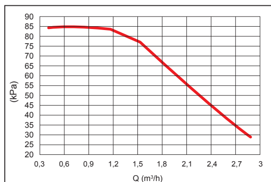
Presión estática externa disponible VS Caudal
