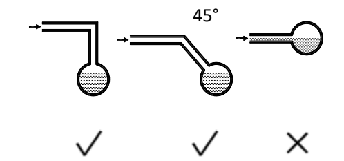
Figura 3-6.3: Tubería de derivación de vaciado que se une a la tubería de vaciado principal
