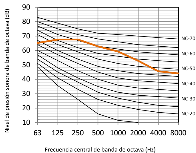
Figura 2-10.10: Nivel de banda de octava de 24 CV
