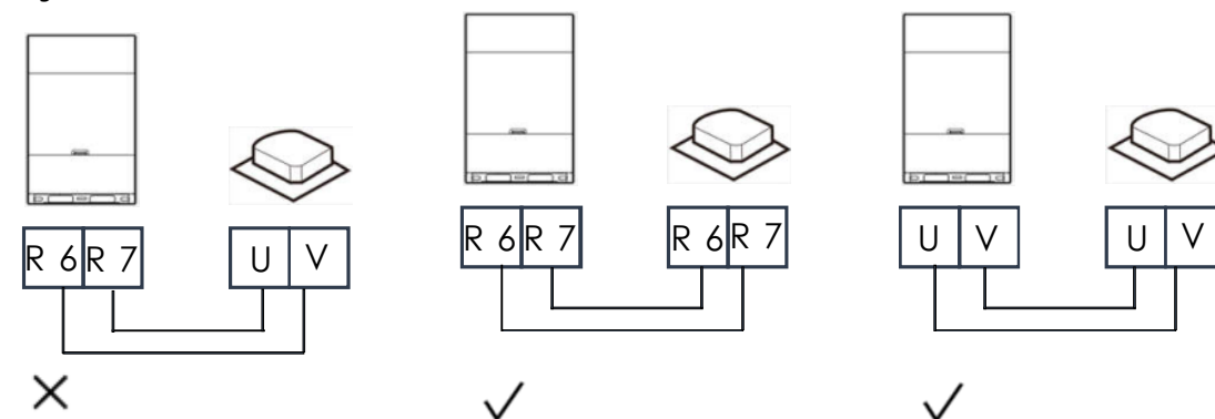
Figura 3-9.5: Cableado de comunicación
