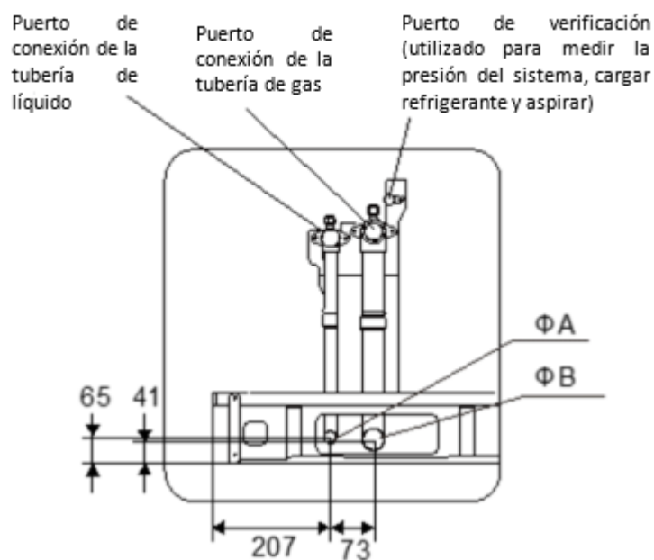
Figura 2-2.4: Detalle R (unidad: mm)
