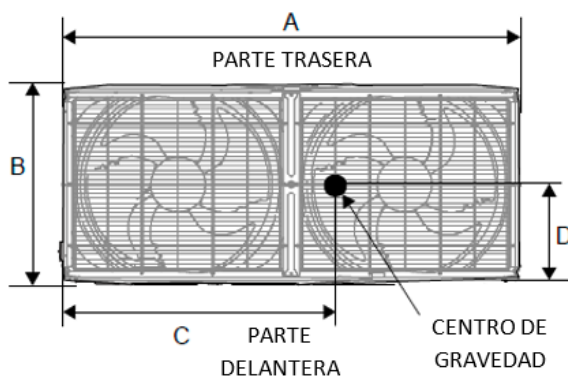
Figura 3-2.9: Centro de gravedad de las unidades de 18-32 CV
