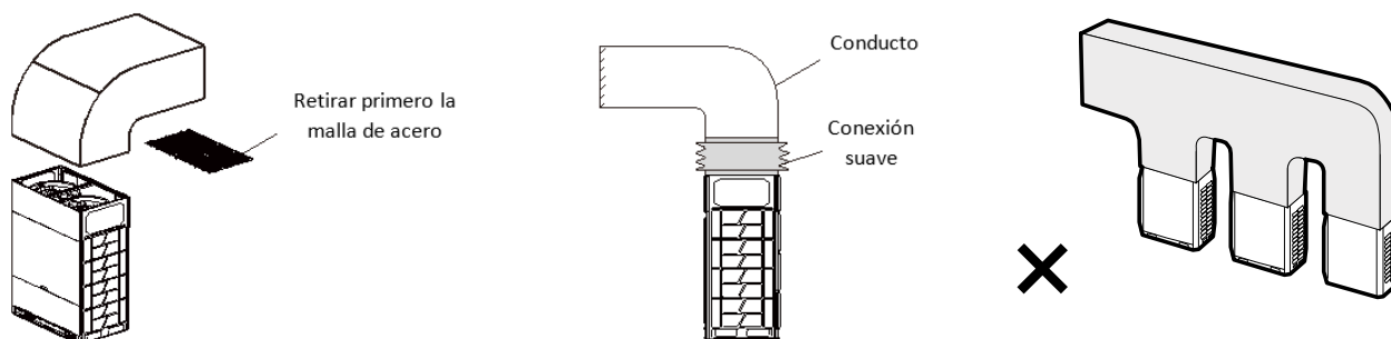
Figura 3-3.2: Requisitos de canalización
