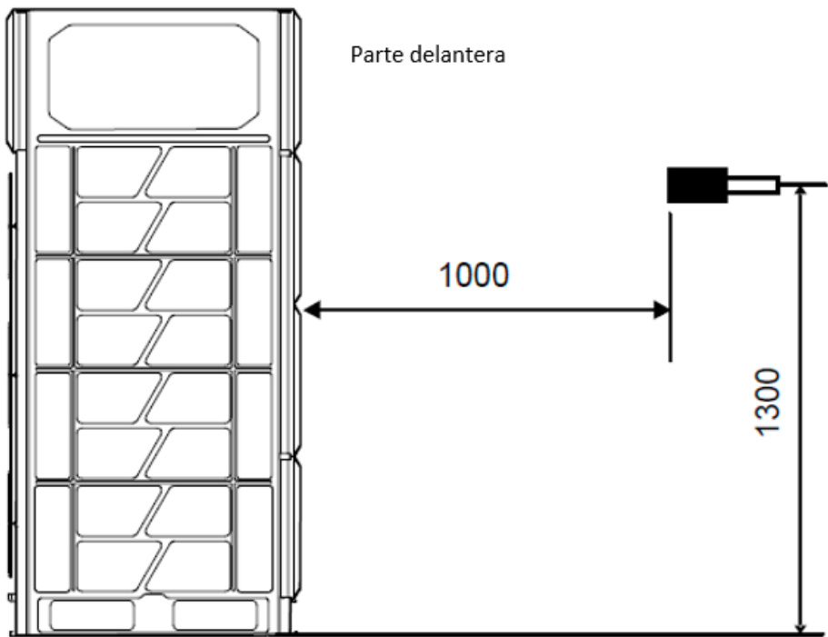
Figura 2-10.1: Medición del nivel de presión sonora (unidad: mm)
