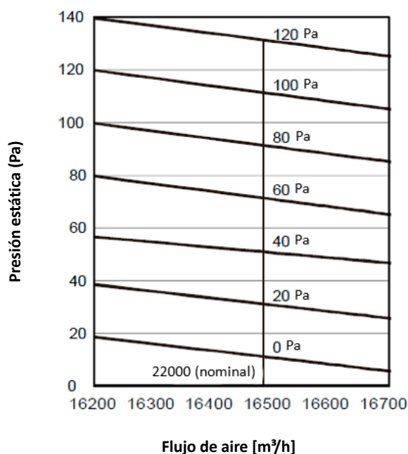
Figura 3-3.7: Rendimiento del ventilador de unidades de 20-24 CV
