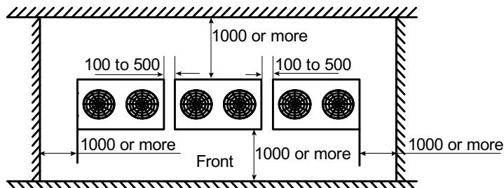
Figura 3-2.2: Instalación de una fila (unidad: mm)
