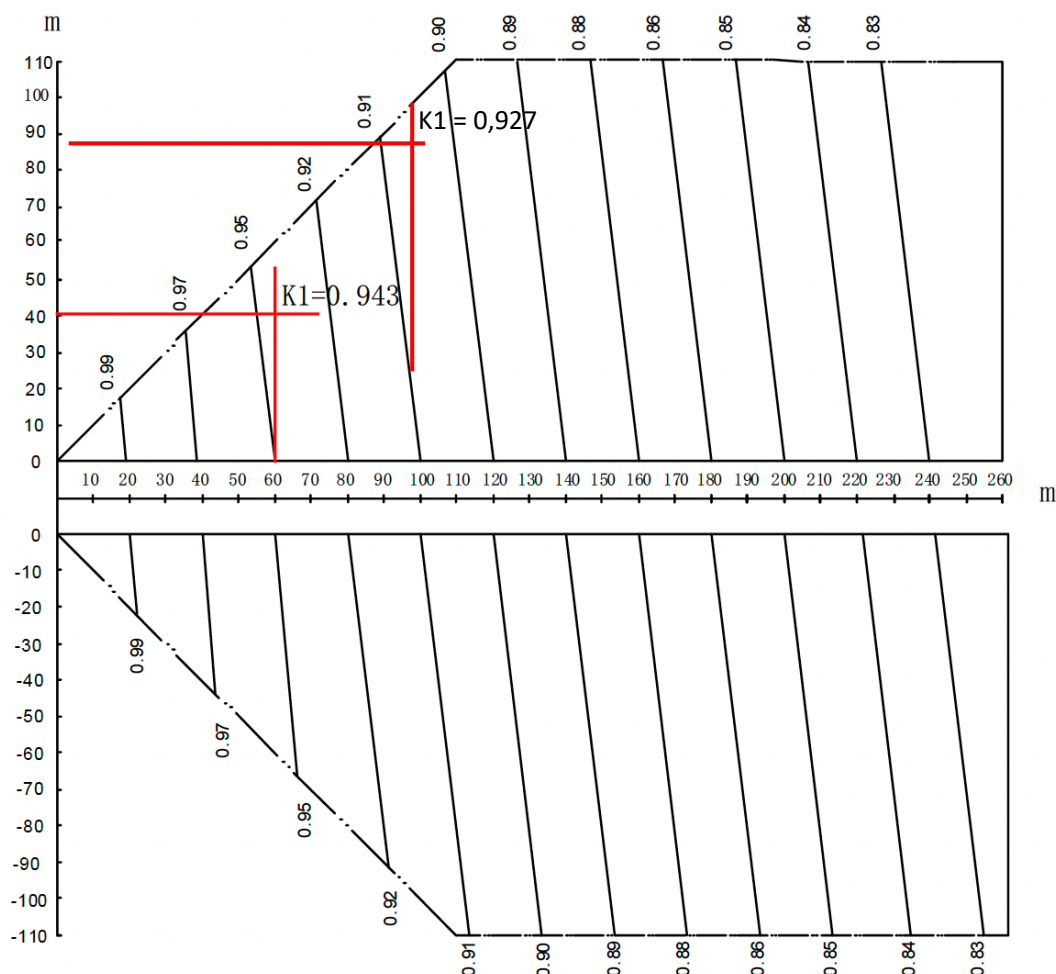
Figura 1-6.3: Tasa de cambio en la capacidad de refrigeración de V8i
