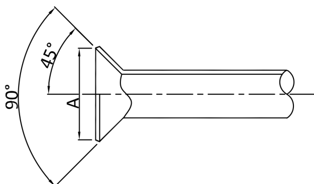
Figura 3-5.2: Apertura abocardada
