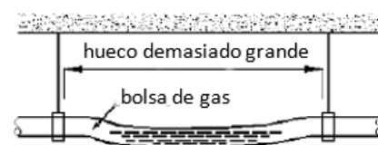
Figura 3-6.4: Efecto de un soporte insuficiente de la tubería de vaciado
