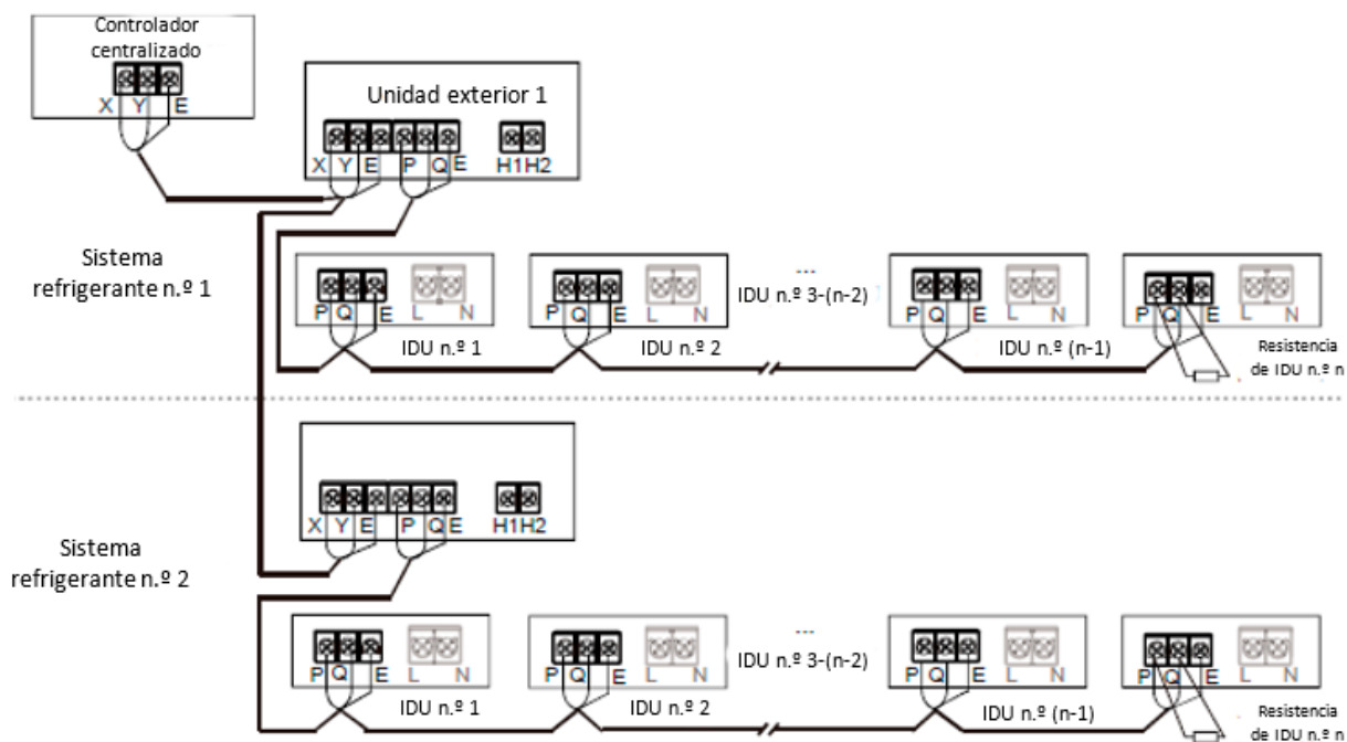
Figura 3-9.12: Comunicación para unidades exteriores
