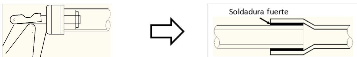
Figura 3-5.1: Extremos de tuberías de cobre expandibles
