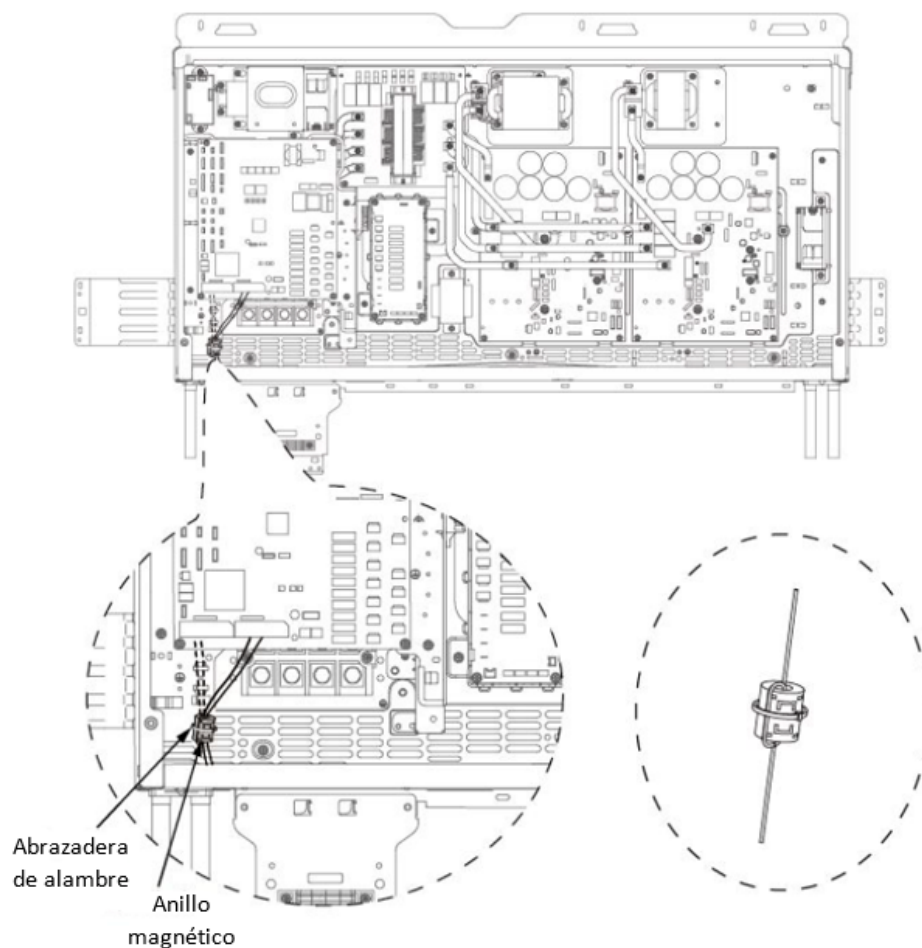
Figura 3-9.6: Instalación del anillo magnético
