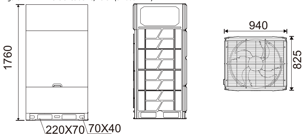
Figura 2-2.1: Dimensiones de 10/16 CV (unidad: mm)
