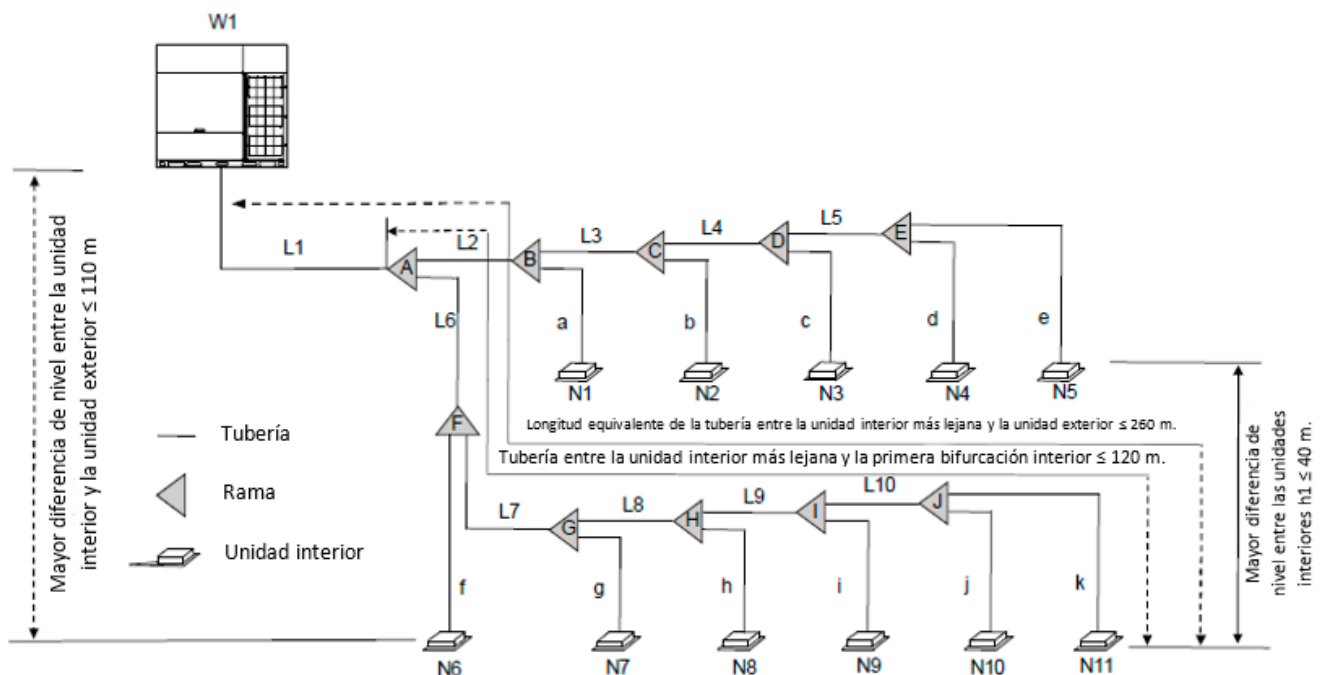
Figura 3-4.1: Longitudes de tuberías de refrigerante y diferencias de nivel permitidas
