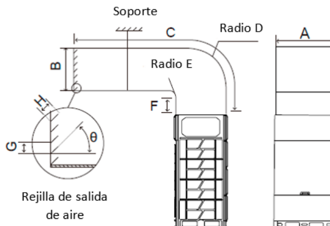
Figura 3-3.3: Conductos transversales (unidad: mm)
