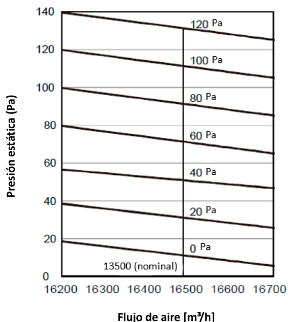
Figura 3-3.7: Rendimiento del ventilador de unidades de 20-24 CV
