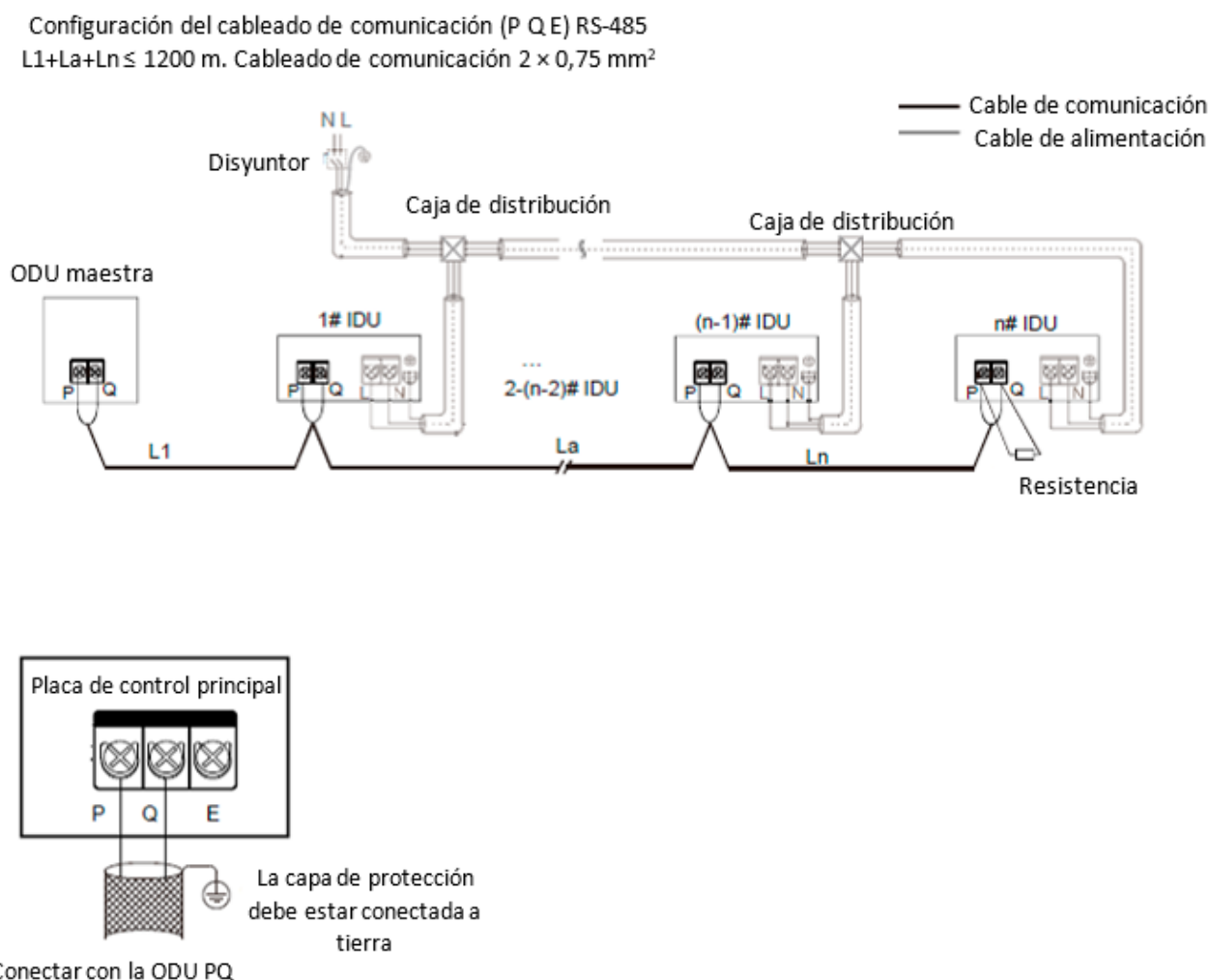
Figura 3-9.8: Configuración del cableado de comunicación P Q: alimentación uniforme de IDU suministrada
