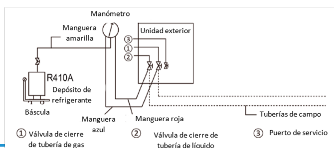
Figura 3-8.1: Carga de refrigerante
