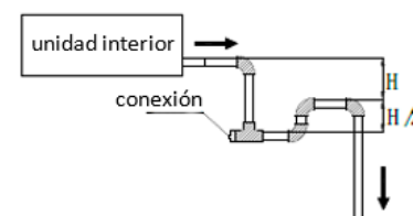
Figura 3-6.6: Trampillas de agua para tuberías de vaciado
