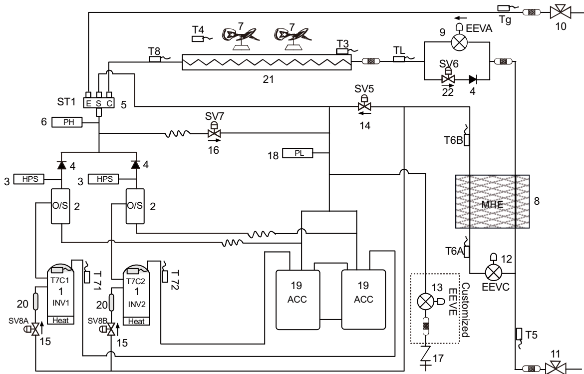
Figura 2-4.3: Diagrama de tuberías de 28-32 CV
