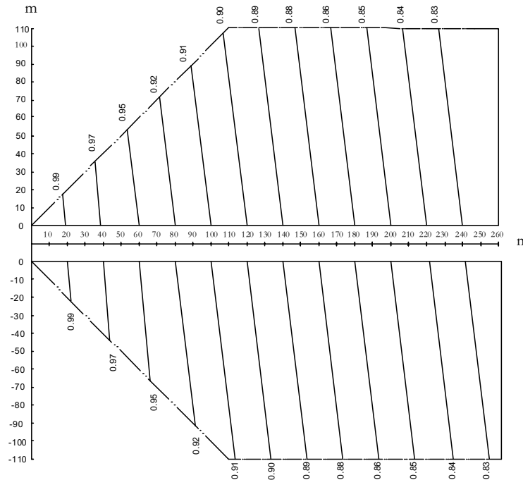
Figura 2-8.2: Tasa de cambio en la capacidad de calefacción
