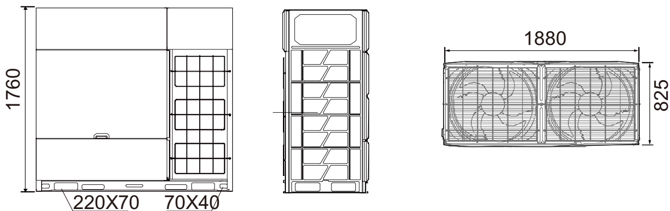
Figura 2-2.3: Dimensiones 28/32 CV (unidad: mm)
