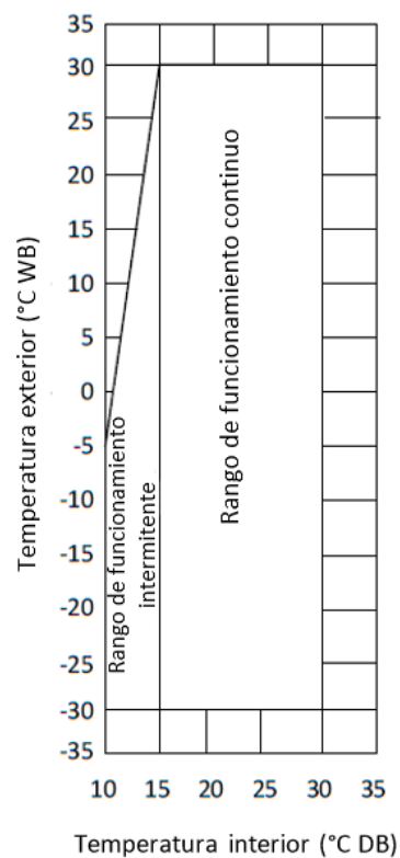
Figura 2-9.2: Límites de funcionamiento de la calefacción
