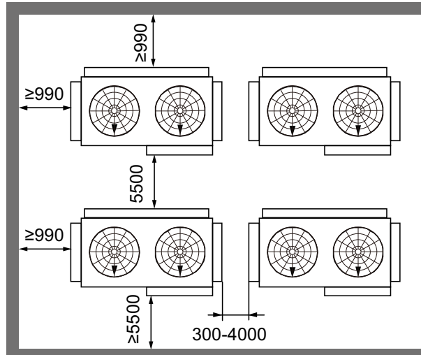
Figura 3-3.10: Instalación de las ODU en dos filas (unidad: mm)
