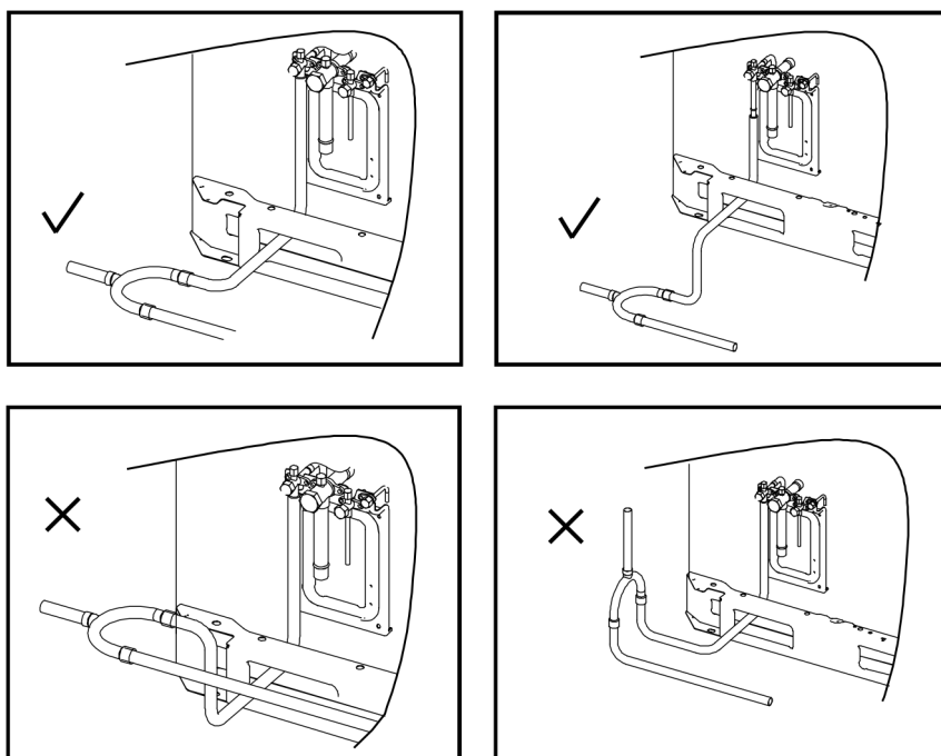
Figura 3-5.9: Instalación de derivaciones exteriores
