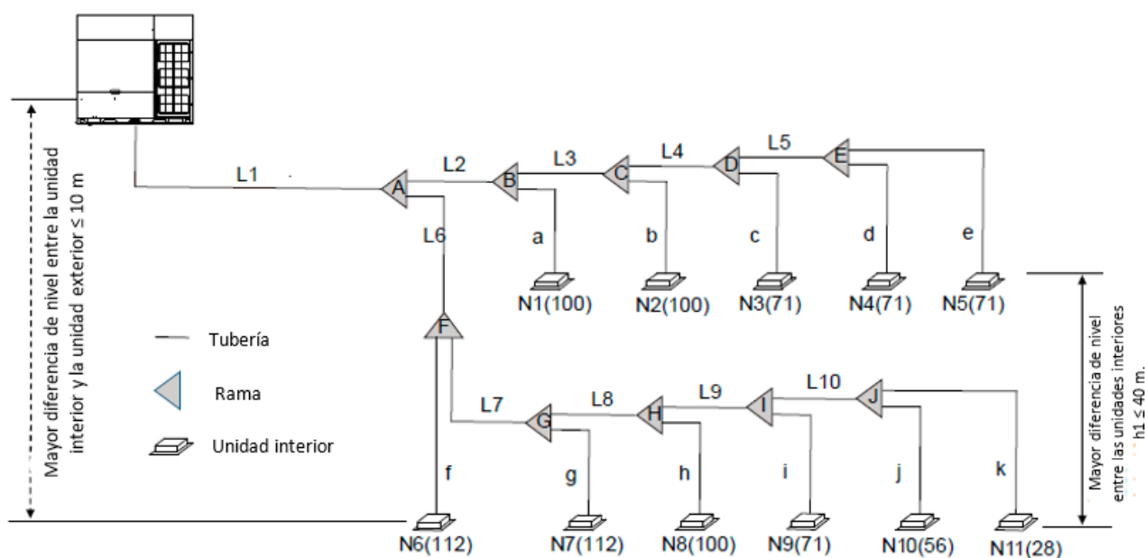
Figura 3-4.5: Ejemplo de selección de tuberías de refrigerante
