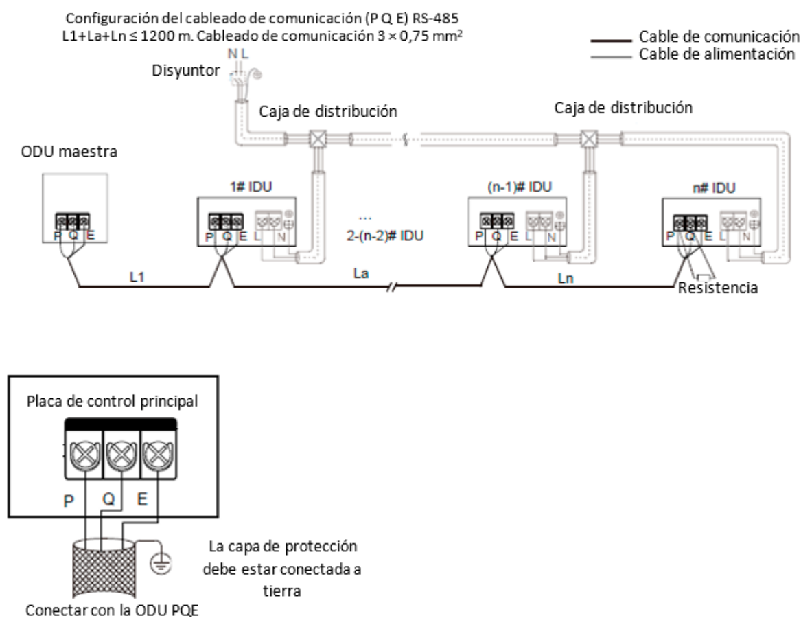
Figura 3-9.7: Configuración del cableado de comunicación P Q E: alimentación uniforme de IDU suministrada
