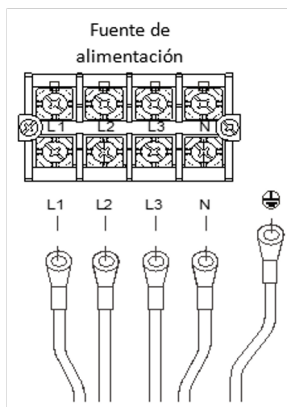
Figura 3-9.4: Terminales de la fuente de alimentación trifásica de la unidad exterior
