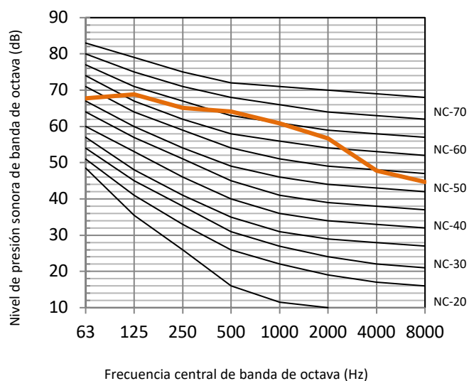
Figura 2-10.14: Nivel de banda de octava de 32 CV
