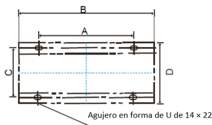
Figura 3-2.3: Ubicación del perno de expansión
