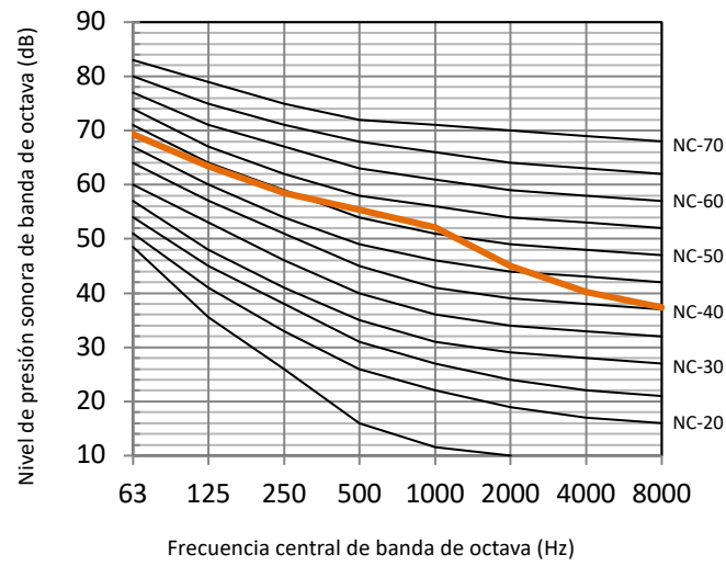
Figura 2-10.3: Nivel de banda de octava de 10 CV
