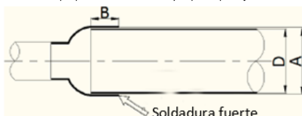
Figura 3-5.7: Superposición de tuberías y espacio para juntas soldadas
