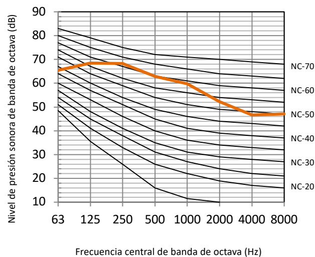
Figura 2-10.8: Nivel de banda de octava de 20 CV
