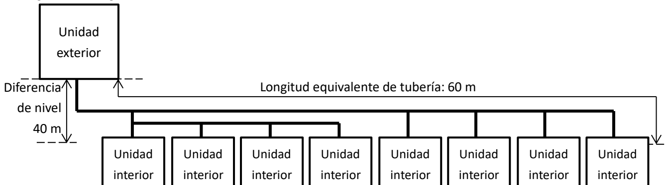
Figura 1-6.2: Diagrama del sistema
