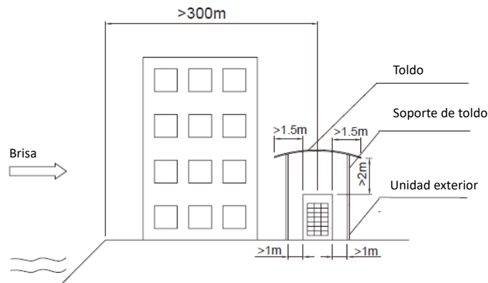
Figura 3-10.2: Instalación en exterior bajo un toldo
