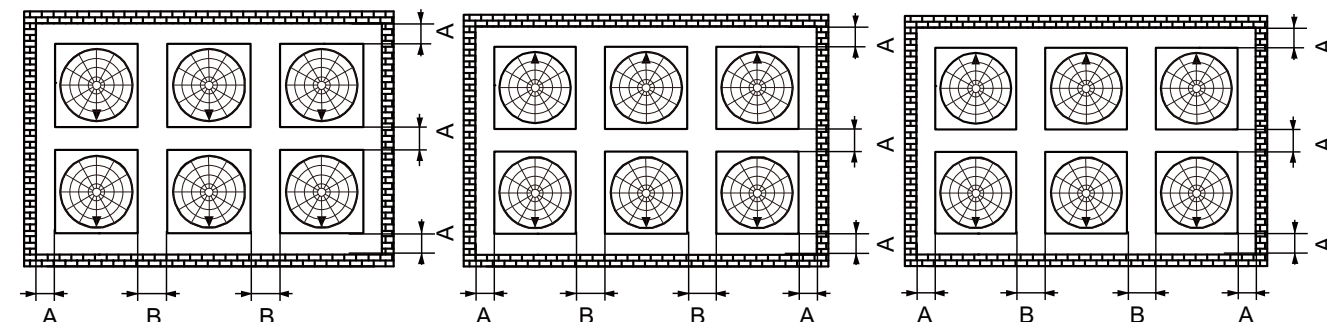
Figura 2-3.4: Instalación con paredes en cuatro direcciones (unidad: mm)
