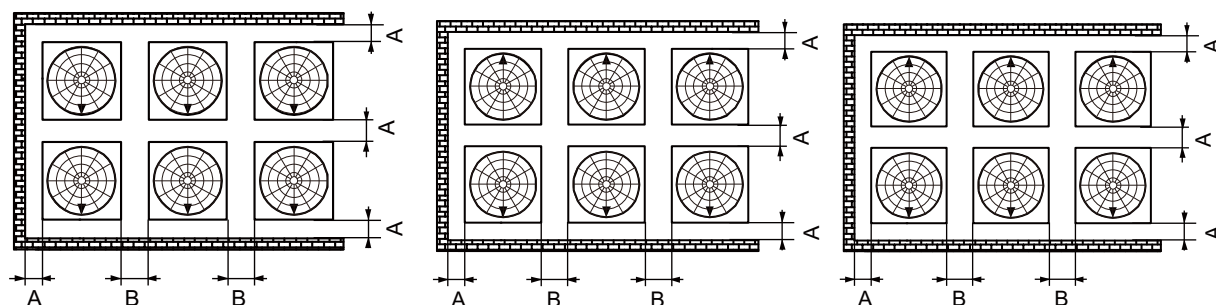
Figura 2-3.3: Instalación con paredes en tres direcciones (unidad: mm)
