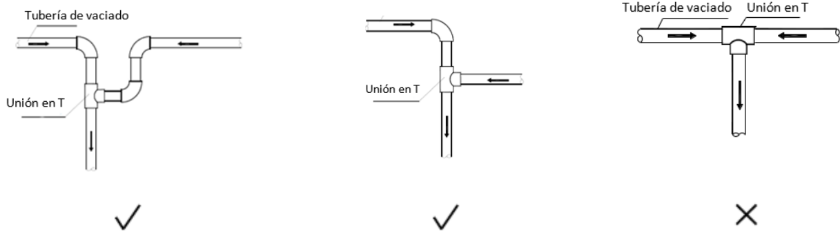
Figura 3-6.3: Tubería de derivación de vaciado que se une a la tubería de vaciado principal
