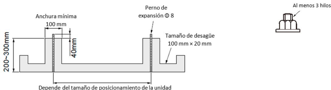
Figura 3-2.2: Diseño típico de estructura de base de hormigón de la unidad exterior (unidad: mm)
