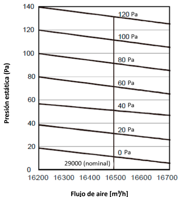
Figura 3-3.8: Rendimiento del ventilador de unidades de 28-32 CV
