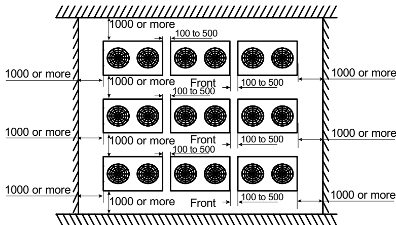
Figura 3-2.3: Instalación en varias filas (unidad: mm)
