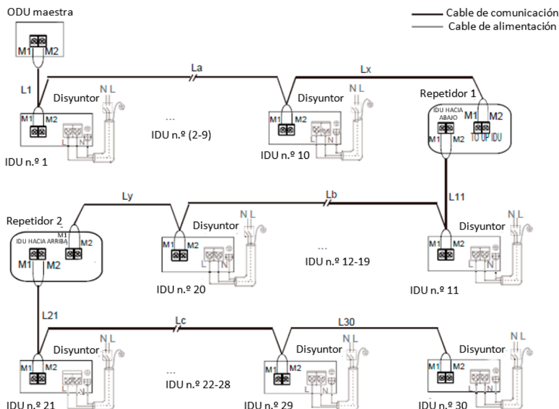
L1+La+Lx \leq 200 m, L11+Lb+Ly \leq 200 m, L21+Lc+L30 \leq 200 mm. Cableado de comunicación 2 \times 1,5 mm 2
