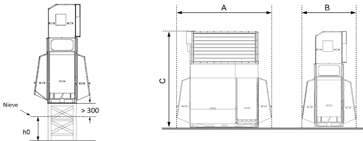
Figura 3-3.9: Protección contra la nieve de la unidad exterior
