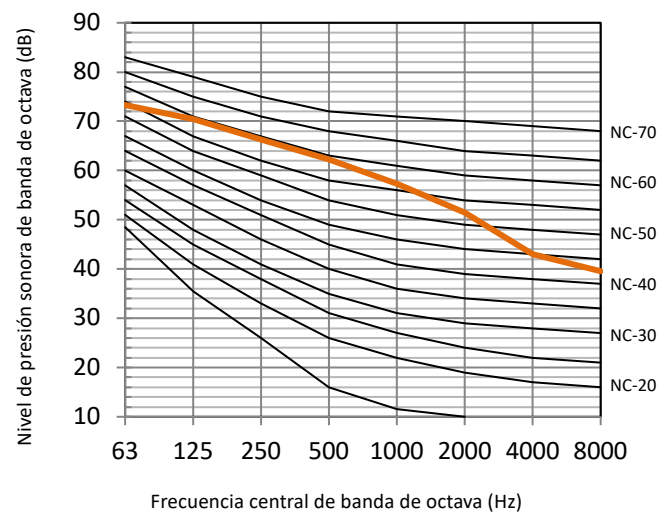
Figura 2-10.6: Nivel de banda de octava de 16 CV
