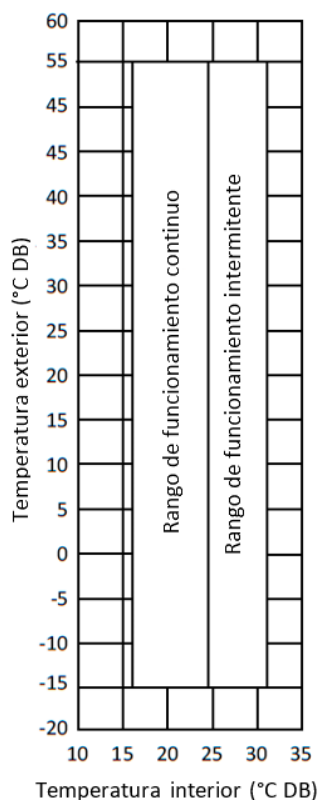
Figura 2-9.1: Límites de funcionamiento de la refrigeración
