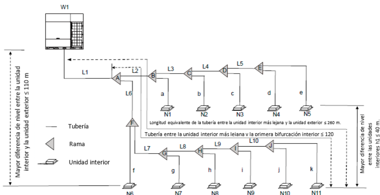
Figura 3-4.3: Selección de diámetros de tuberías
