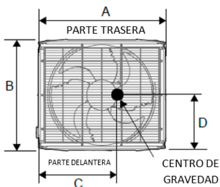
Figura 3-2.9: Centro de gravedad de las unidades de 18-32 CV
