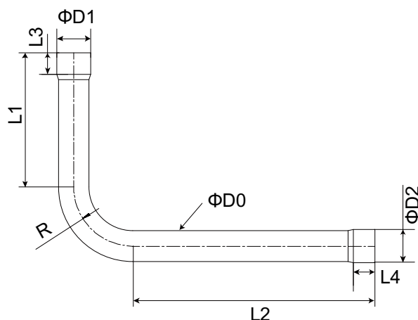
Figura 2-11.2: Tamaño de tubería en forma de L (unidad: mm)
