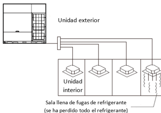
Figura 3-4.7: Escenario potencial de fuga de refrigerante
