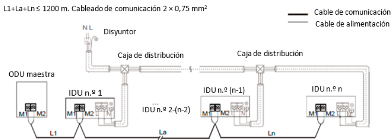
Figura 3-9.9: Configuración del cableado de comunicación M1 M2: alimentación uniforme de IDU suministrada
