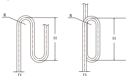
Figura 3-4.2: Codo de retorno de aceite
