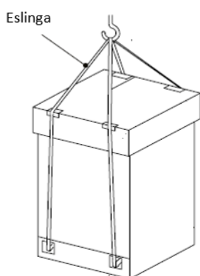
Figura 3-2.4: Elevación
