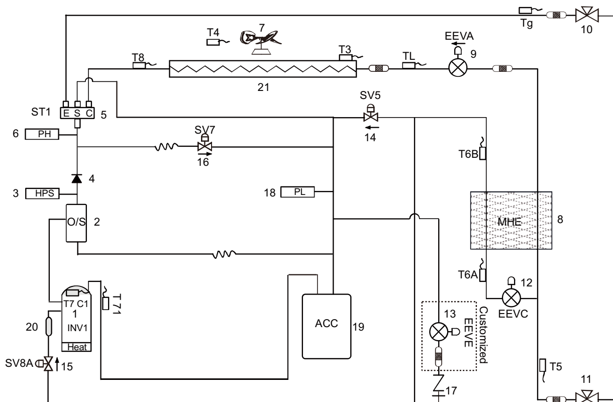
Figura 2-4.1: Diagrama de tuberías de 10-18 CV
