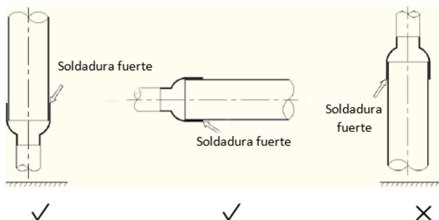
Figura 3-5.6: Orientación de las tuberías durante la soldadura
