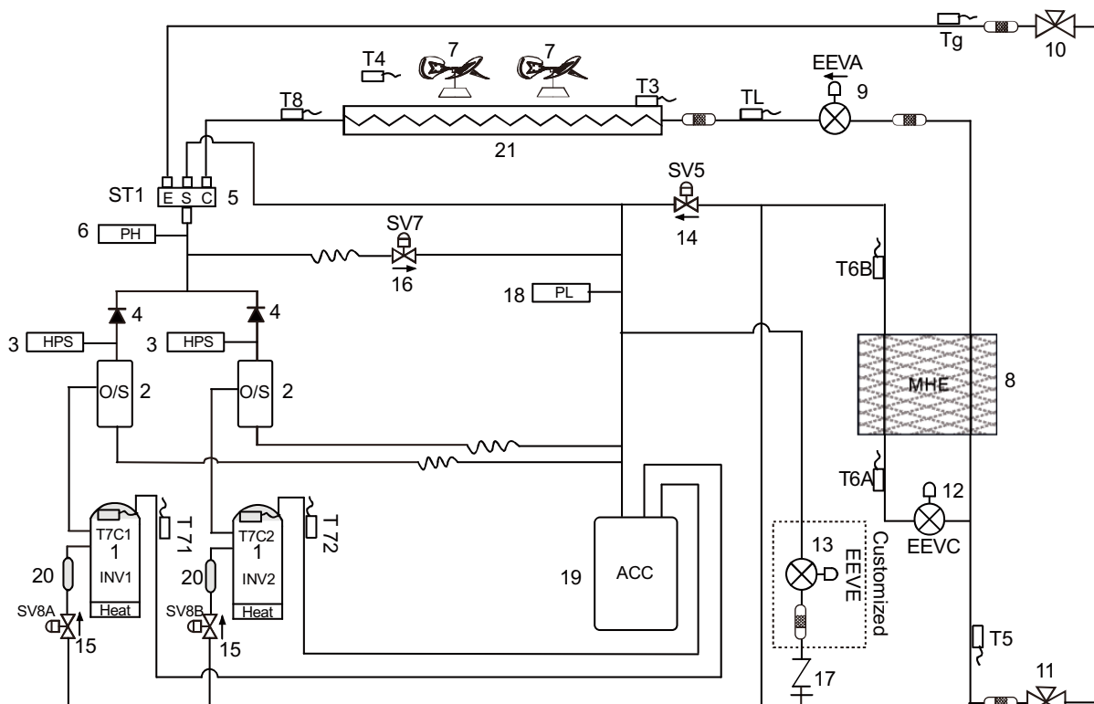
Figura 2-4.2: Diagrama de tuberías de 20-24 CV
