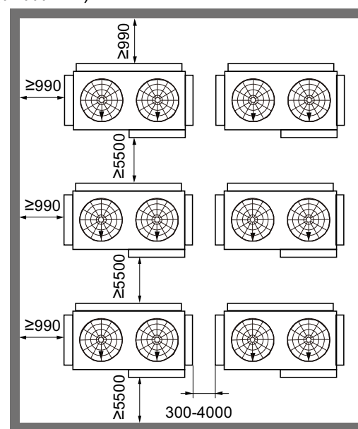
Figura 3-3.10: Instalación de las ODU en dos filas
