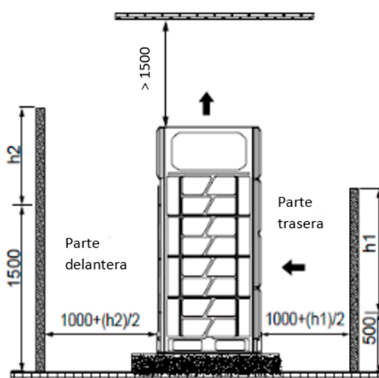
Figura 3-3.1: Parte superior de la unidad por debajo de la parte superior de la unidad de pared adyacente (mm)
