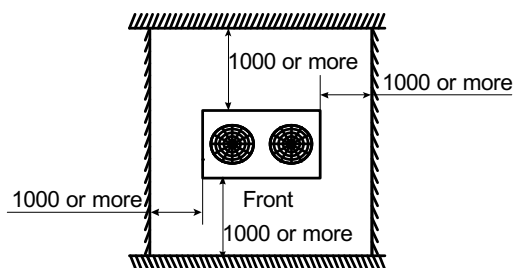
Figura 3-2.1: Instalación de una sola unidad (unidad: mm)
