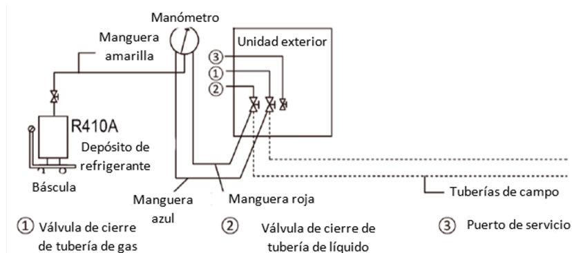
Figura 3-5.15: Secado al vacío
