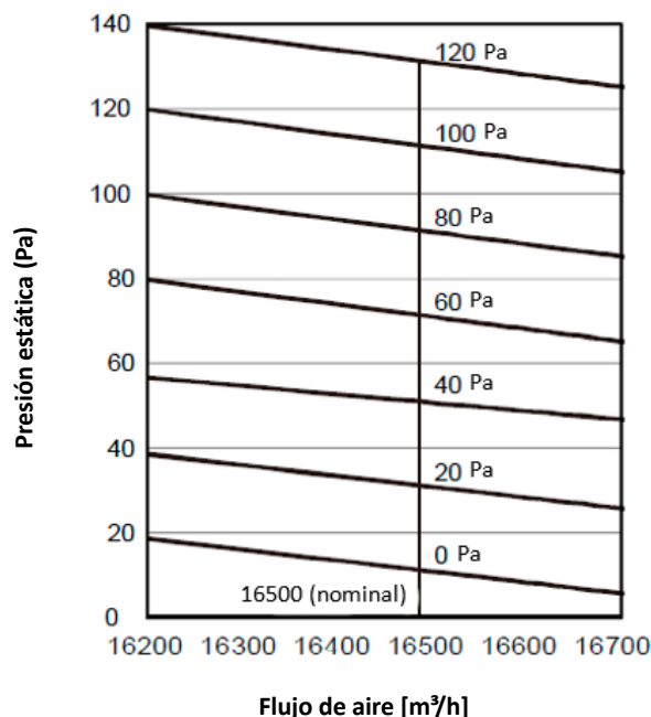
Figura 3-3.6: Rendimiento del ventilador de unidades de 16-18 CV
