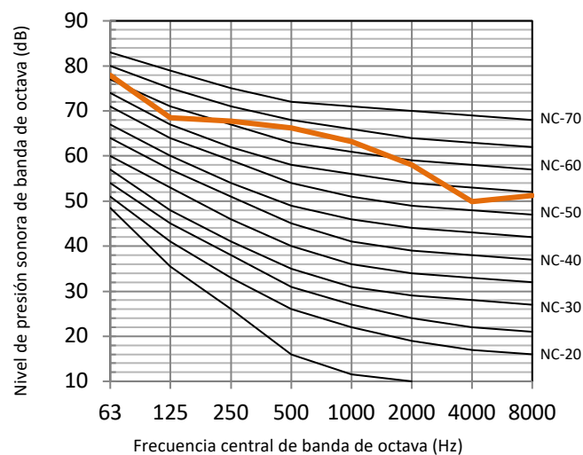
Figura 2-10.12: Nivel de banda de octava de 28 CV
