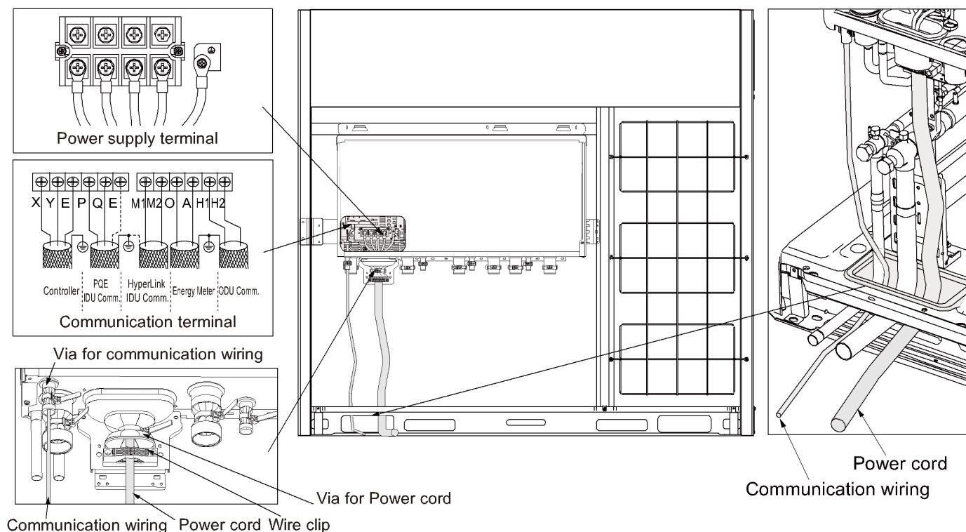
Figura 3-9.1: Diseño del cableado
