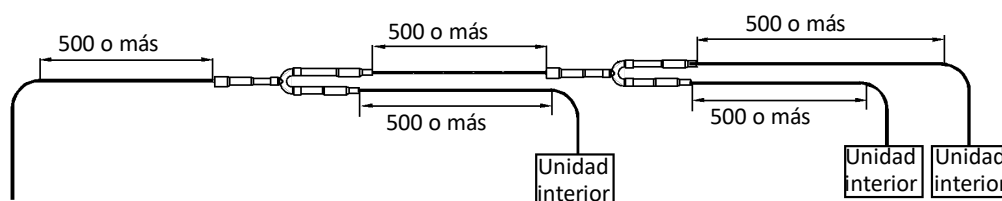
Figura 3-4.6: Separación de los derivadores y separación respecto de las curvas (unidad: mm)
