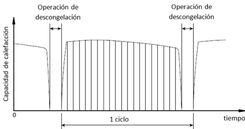
Figura 2-8.3: Ciclo de descongelación
