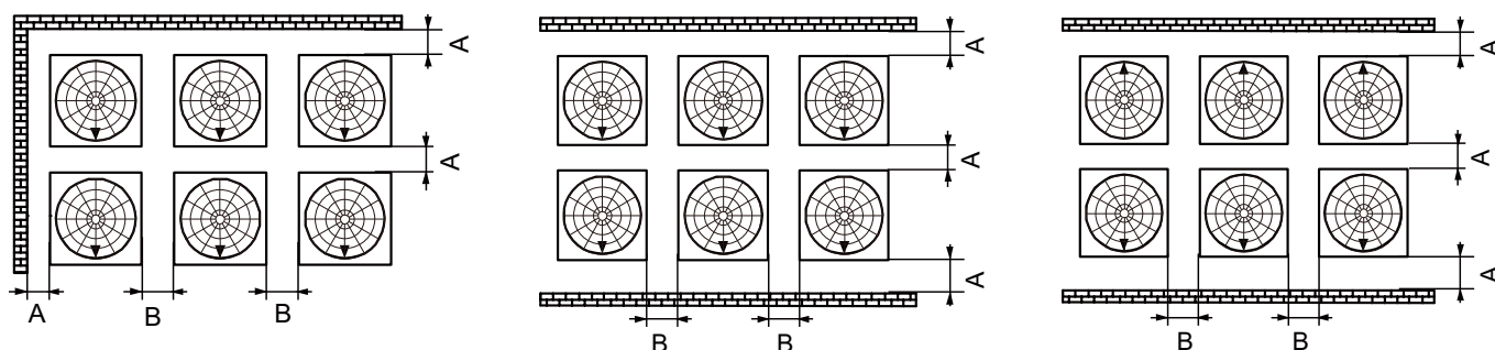
Figura 2-3.2: Instalación con paredes en dos direcciones (unidad: mm)
