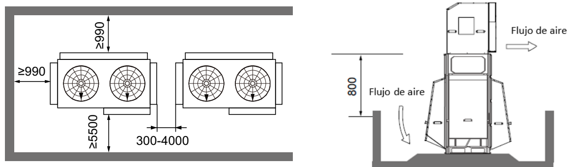
Figura 3-3.10: Instalación de las ODU en fila (unidad: mm)
