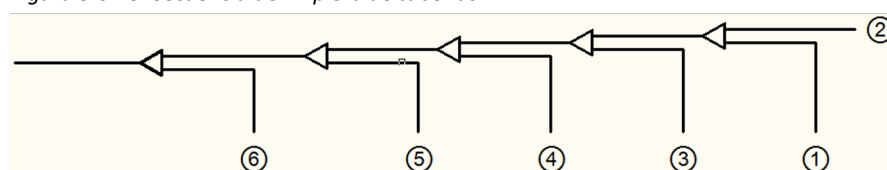
Figura 3-5.13: Secuencia de limpieza de tuberías 1
