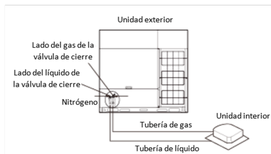
Figura 3-5.14: Prueba de estanqueidad a los gases
