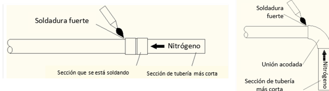
Figura 3-5.5: Flujo de nitrógeno desde el lado más corto durante la soldadura
