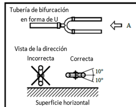
Figura 3-5.8: Orientación de el derivador
