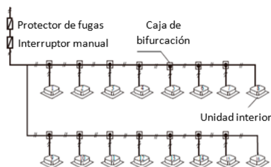
Figura 3-9.3: Cableado de la fuente de alimentación de la unidad interior
