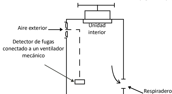
Figura 3-4.8: Ventilador mecánico controlado mediante detector de fugas de refrigerante
