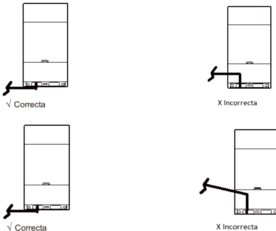
Figura 3-5.10: Conexiones de tuberías de la unidad exterior
