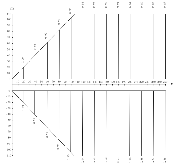
Figura 2-8.2: Tasa de cambio en la capacidad de calefacción
