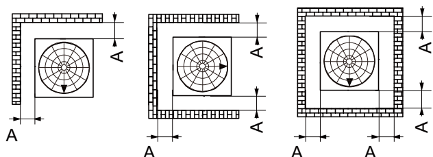
Figura 2-3.1: Instalación de una sola unidad (unidad: mm)
