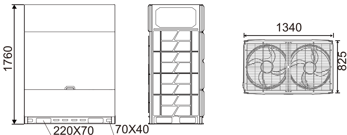
Figura 2-2.2: Dimensiones 20/24 CV (unidad: mm)
