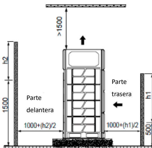
Figura 2-3.5: Parte superior de la unidad por debajo de la parte superior de la unidad de pared adyacente (mm)
