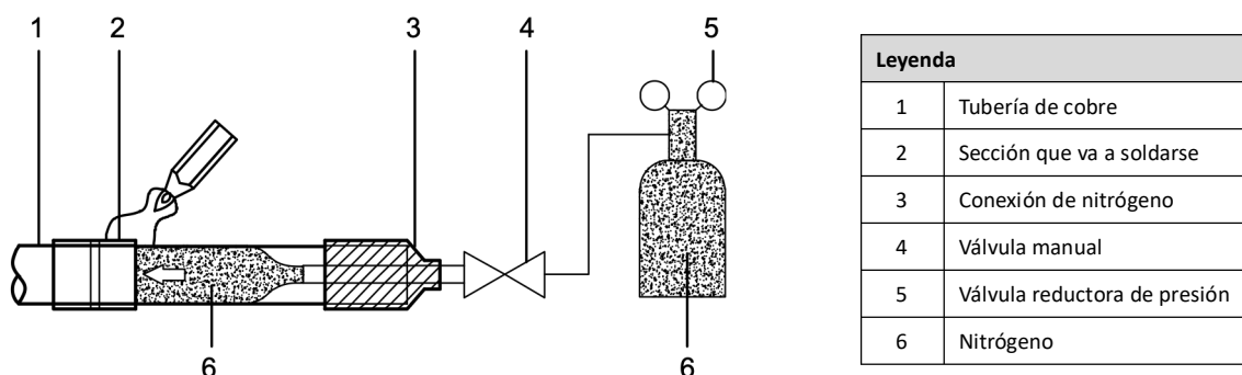
Figura 3-5.4: Flujo de nitrógeno a través de las tuberías durante la soldadura
