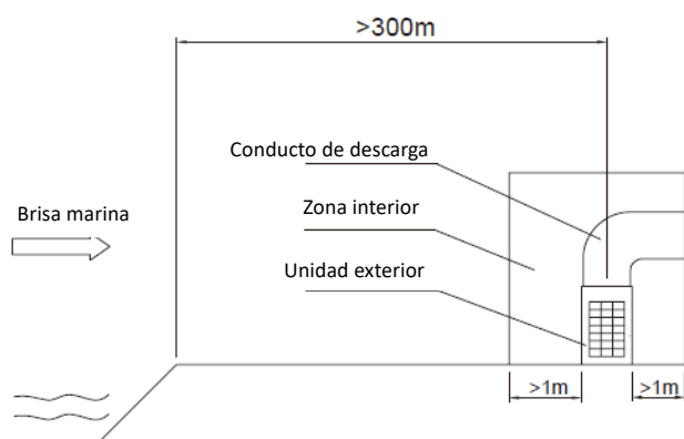
Figura 3-10.1: Instalación en un zona interior bien ventilada
