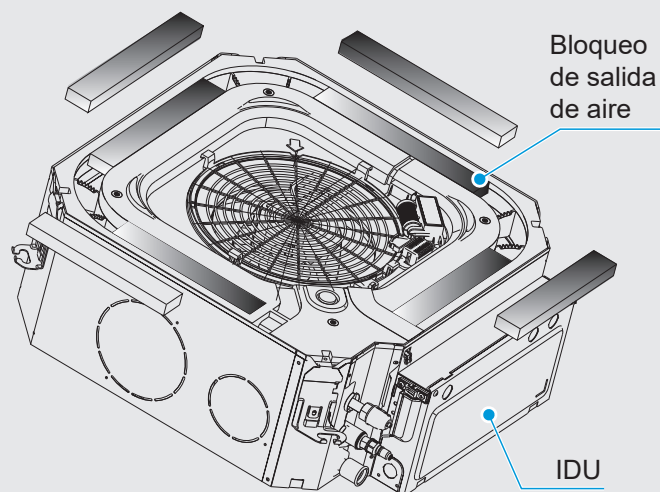
Esquema de una salida de aire bloqueada
