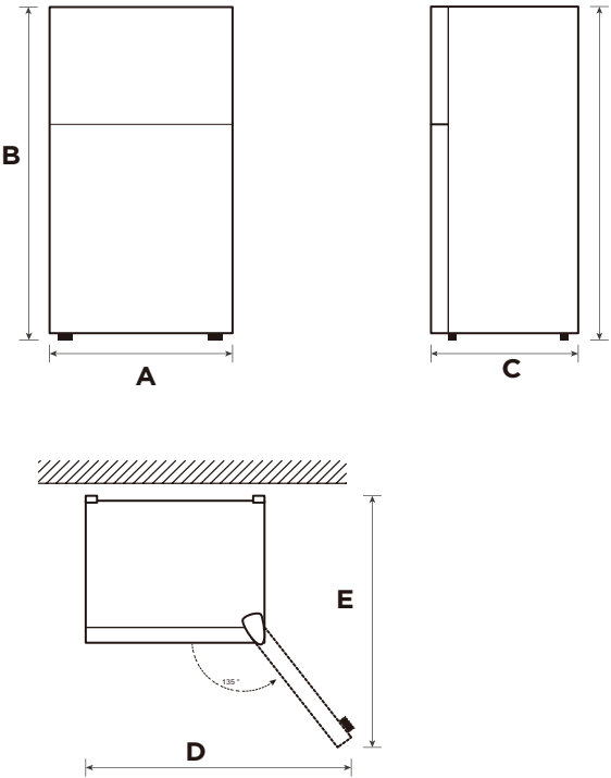
Diagramm zum Freiraumbedarf (bei geöffneter und geschlossener Tür)
