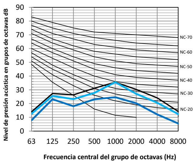
Fig. 7.6: Niveles grupos de octavas HRV-D800(C) (KRE D800D2)
