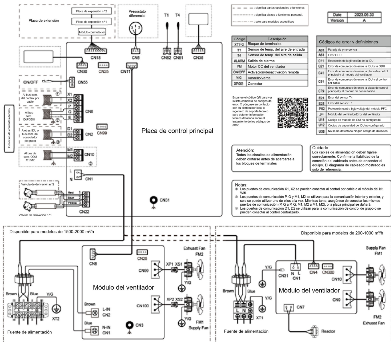
Imagen 5.1: Diagrama de cableado del HRV
