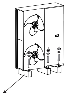
Almohadilla antivibración
